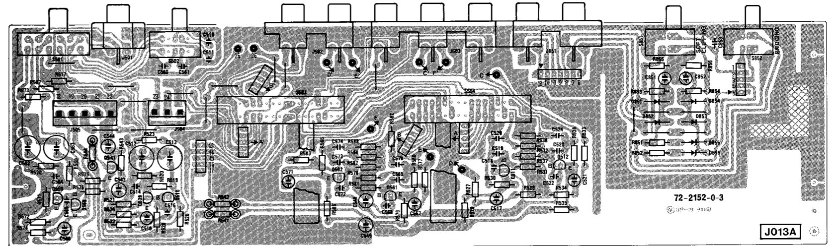
INPUT/OUTPUT PCB
