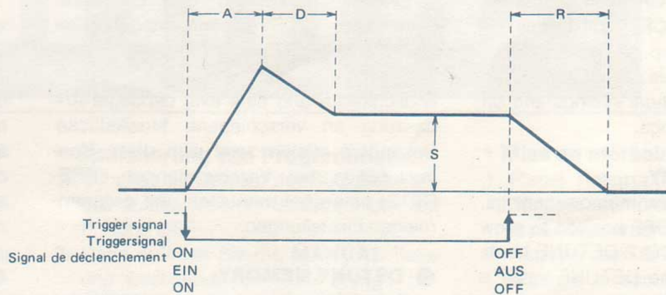
"ADSR"-Hüllkurvensignal
